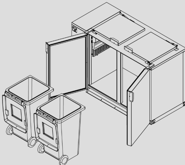
Rys. 4 Pozycja najazdowa koszy (otwarta pokrywa)
