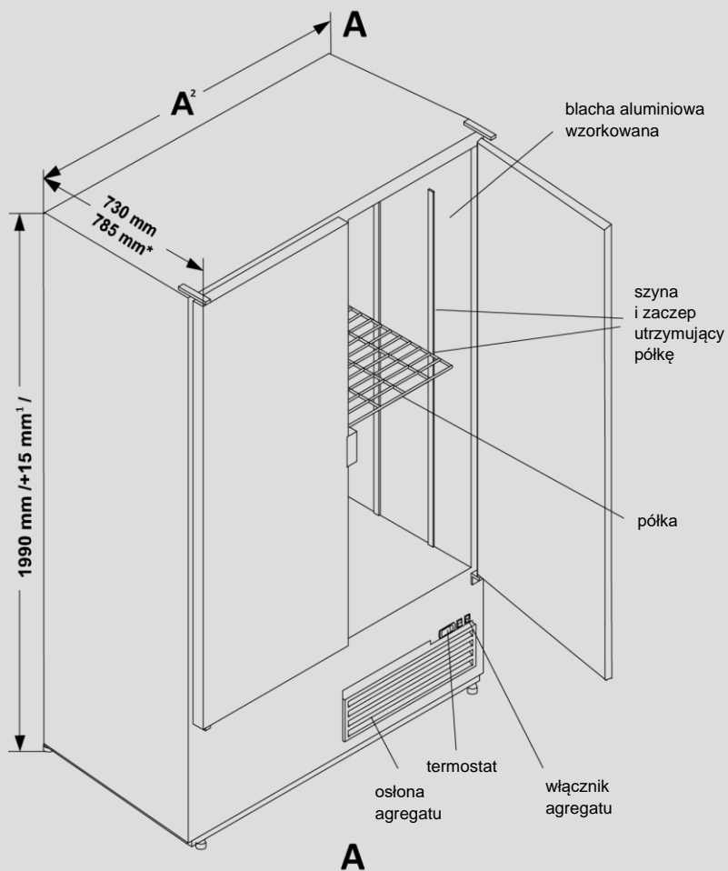
Rys. 1 PRZYKŁADOWY SZKIC IZOMETRII SZAF CHŁODNICZYCH MODELII: Z, ZR, S, SR, 2S, 2S/1D, 2SR, 2SR/1D, 2S2R
