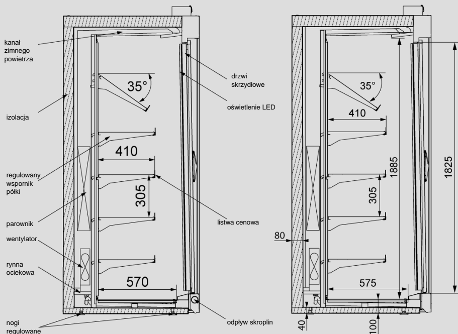
Rys. 3 Przekrój regału RCh-GT
