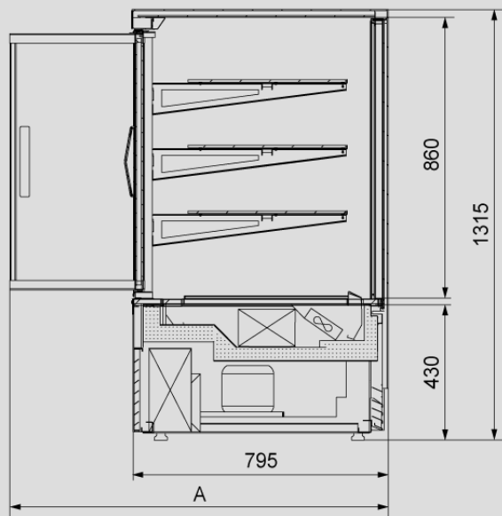
Rys. 1c. przekrój poprzeczny urządzenia C-C SL EXCELLENTE z drzwiami skrzydłowymi – wymiary gabarytowe
