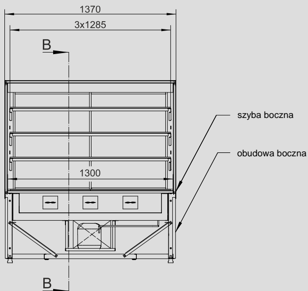
Rys. 4. Przekrój wzdłużny – wymiary gabarytowe
