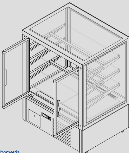
Rys. 2. Izometria
