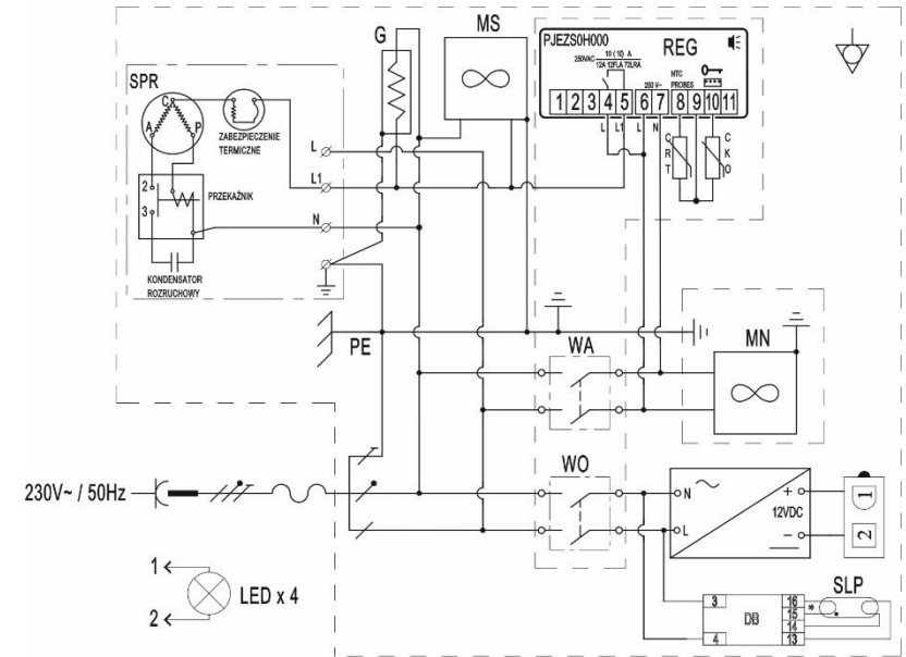
Schemat instalacji elektrycznej witrzyn chłodniczych cukierniczych C-...
