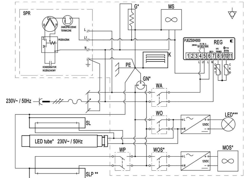
Schemat instalacji elektrycznej ład chłodniczych L-A, A1, A2, A3, B, B1, B2, B3, C, D, D3
