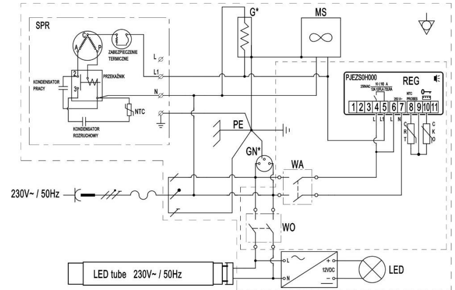
Schemat instalacji elektrycznej ląd chłodniczych L-E, E Max, F, F Max, H, H Max
