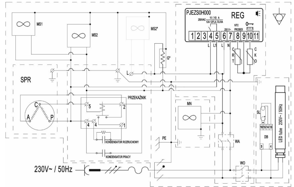
Schemat instalacji elektrycznej regałów chłodniczych RCh...
