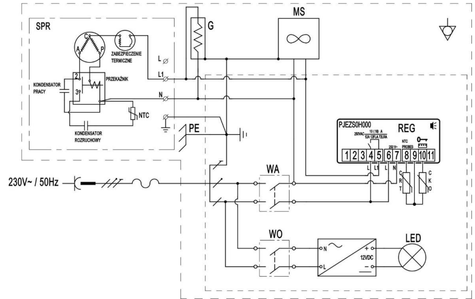
Schemat instalacji elektrycznej altany kwiatowej SCh-AK
