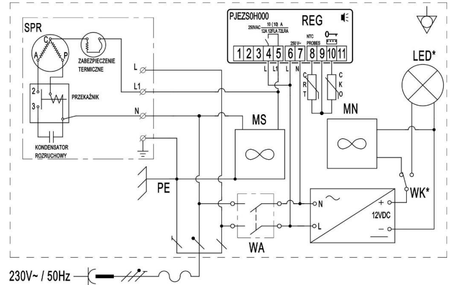
Schemat instalacji elektrycznej szafy SCh-Z, ZR... z wentylatorem nawiewu.
