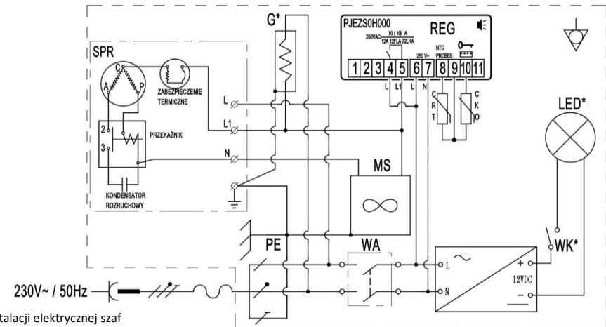
Schemat instalacji elektrycznej szafy chłodniczych modele: SCh-Z, ZR
