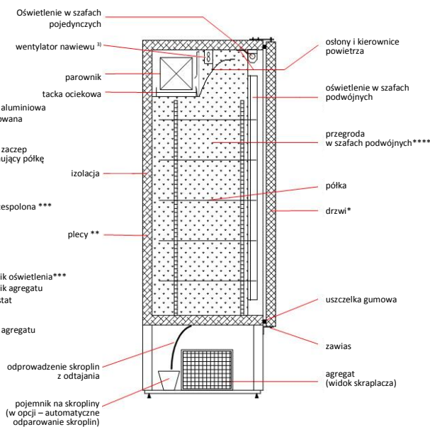
Rys. 2 (przekrój E-E)
